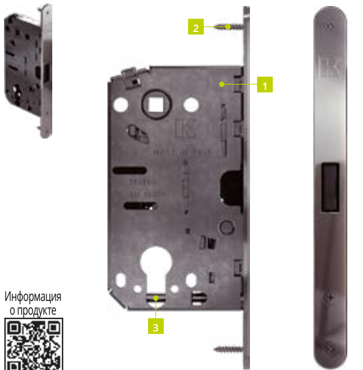
Вид спереди
