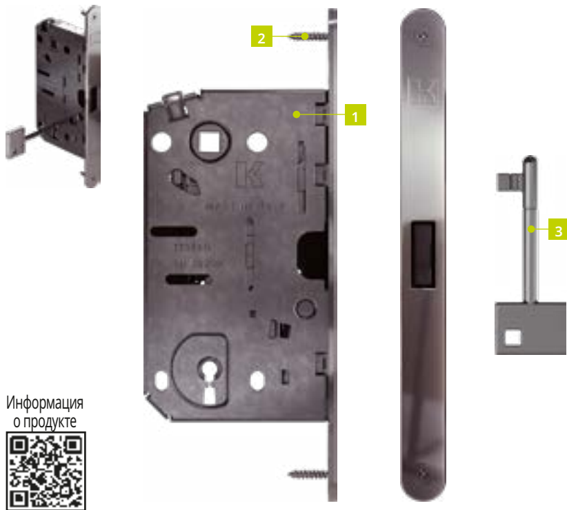
Вид спереди
