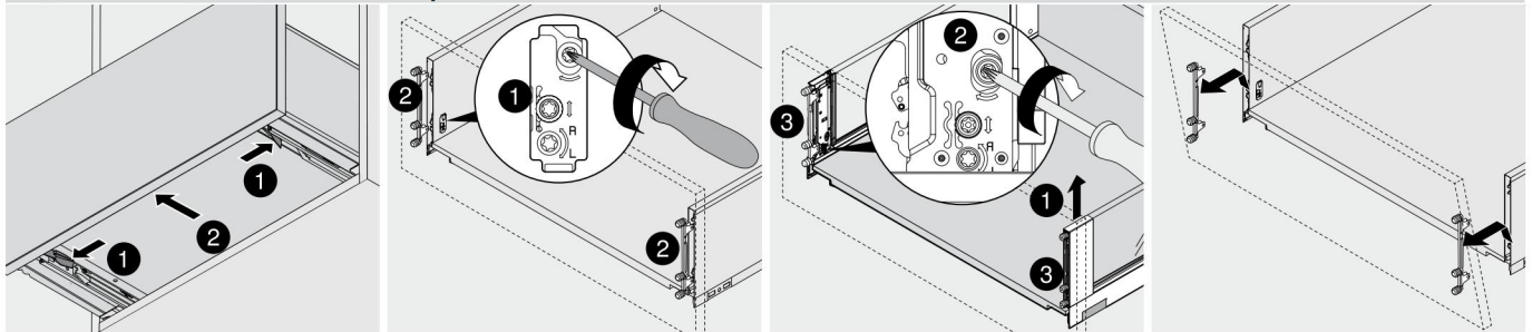
Демонтаж
