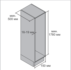
Размеры корпуса
