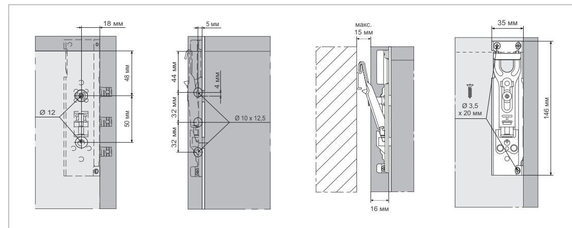
Кронштейн
