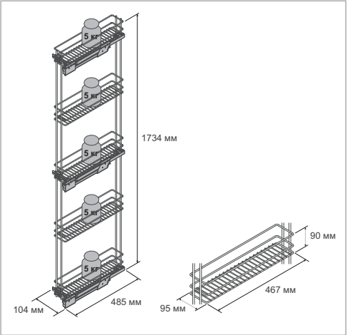
Размеры системы
