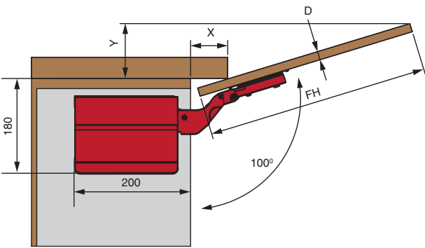
Расчет для установки с карнизом
