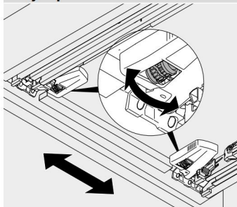
Регулировка по ширине С двух сторон на замках ±1.5 мм
