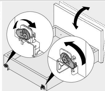
Регулировка наклона
