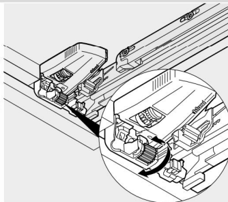
Регулировка по глубине Регулировкой по глубине 298.7600 ± 2 мм
