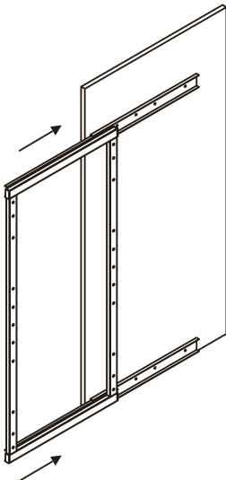
3. Установка несущей рамы
