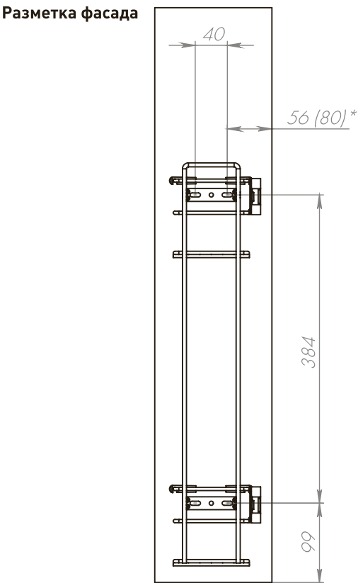
Разметка под направляющие 35 мм
