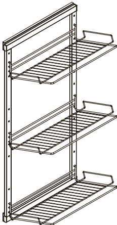
3-х ур. обувница Габаритные размеры (ШхГхВ) 315х480х1015
