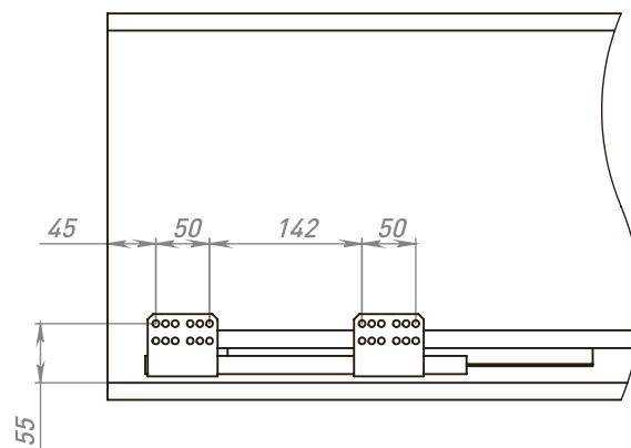
Разметка под направляющие
