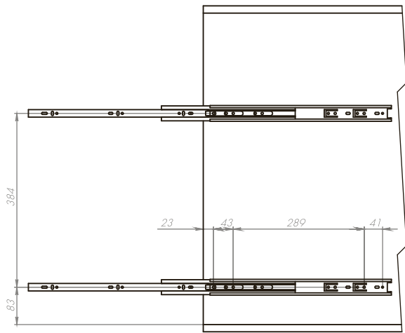
Разметка под направляющие 35 мм
