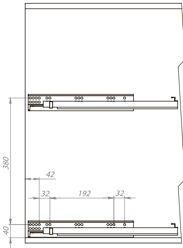
Разметка под направляющие
