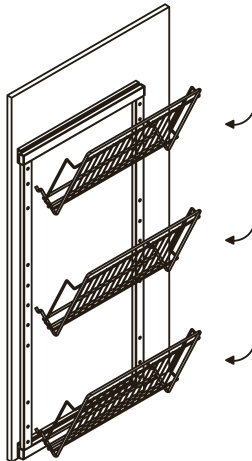
4. Установка корзин на раму
