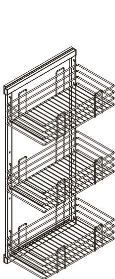
3-х ур. корзина Габаритные размеры (ШхГхВ) 285х475х1015
