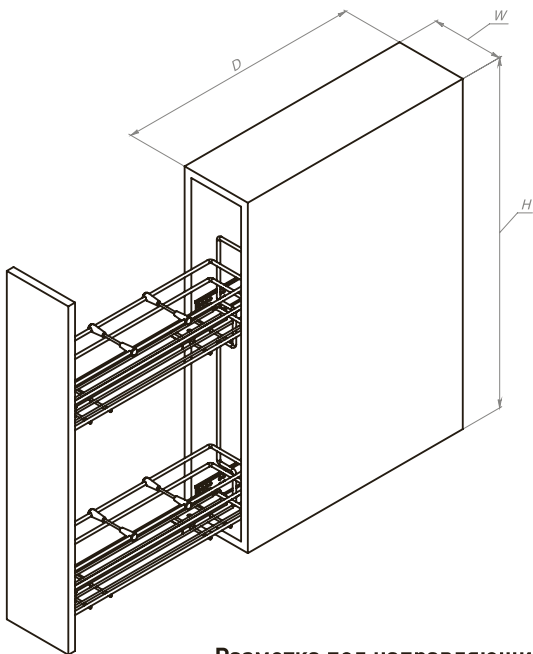
Разметка под направляющие
