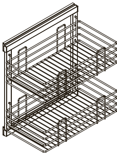
2-х ур. обувница Габаритные размеры (ШхГхВ) 285х475х515
