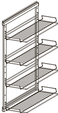
4-х ур. обувница Габаритные размеры (ШхГхВ) 315х480х1015
