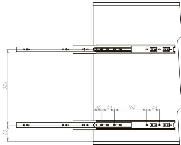
Разметка под направляющие 45 мм
