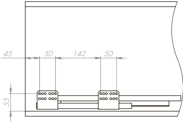
Разметка под направляющие
