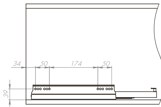
Разметка под направляющие
