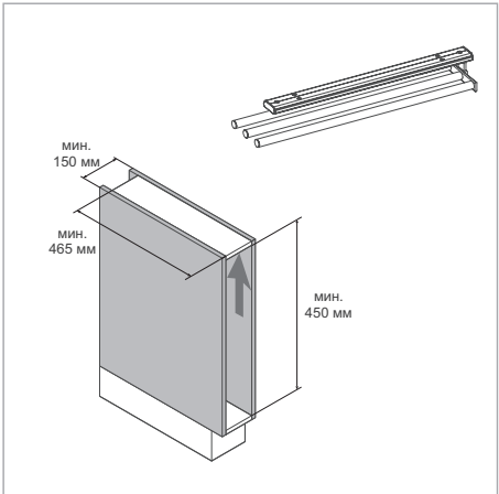
Размеры корпуса при креплении к верхней части
