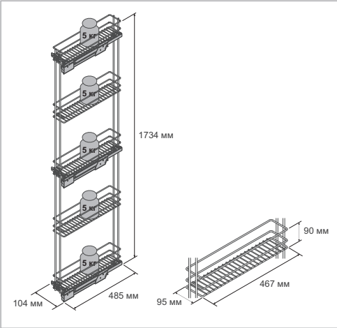
Размеры системы
