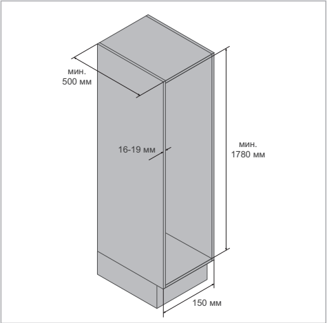
Размеры корпуса
