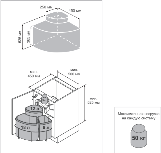
Размеры корпуса и системы с тремя ведрами
