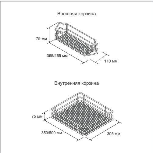
Высота корзины в дизайне Planego 80 мм*
