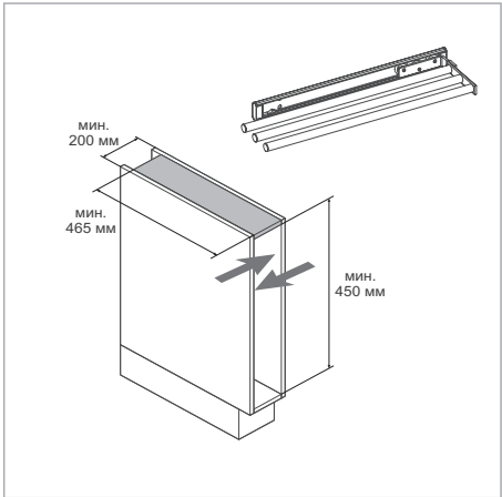
Размеры корпуса при креплении к боковине
