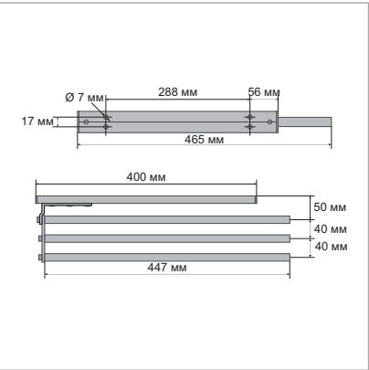
Размеры системы
