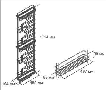
Размеры системы
