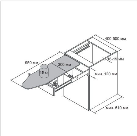
Размеры корпуса и системы
