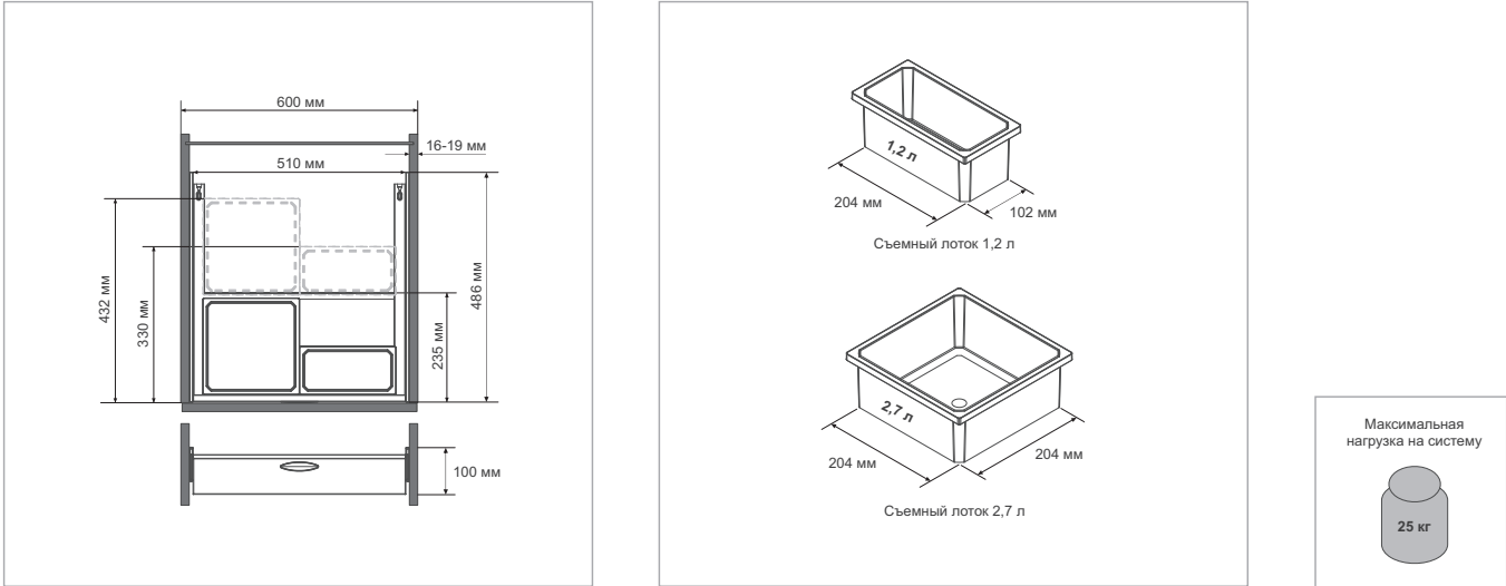
Размеры корпуса и систем
