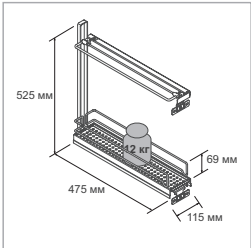
Размеры системы
