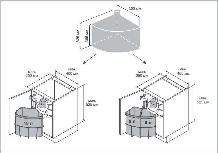
Размеры корпуса и систем с одним и двумя ведрами
